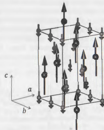
Рис. 12. Магнитная структура \text{DyCo}_2 . Длинные стрелки-момент диспрозия, короткие стрелки-момент кобальта.
