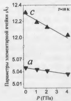
Рис. 19. Барические зависимости параметров элементарной ячейки \text{ErCo}_2 при T = 10 К. Ошибки не превышают размеров символов. Сплошные линии – линейная интерполяция экспериментальных данных.
