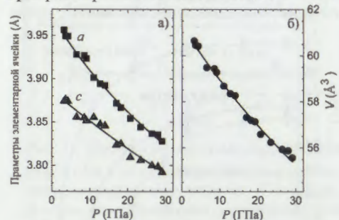
Рис. 7. Барические зависимости параметров (а) и объема элементарной ячейки, интерполированного уравнением Берча – Мурнагана (б) \text{La}_{0,5}\text{Ba}_{0,5}\text{CoO}_{2,8} . Ошибки не превышают размеров символов.
