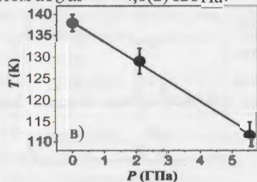
Рис. 13. Температурные зависимости упорядоченных магнитных моментов Со (а) и Ду (б) при различных давлениях. Линии – интерполяция экспериментальных данных функцией (1). Зависимости T_C кобальтовой и диспризиевой подрешёток от давления (в).
