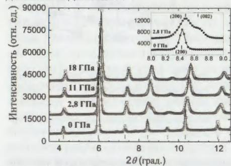
Рис. 6. Участки рентгеновских дифракционных спектров \text{La}_{0,5}\text{Ba}_{0,5}\text{CoO}_{2,8} полученные при различных давлениях и комнатной температуре, обработанные по методу Ритвельда. На вставке представлено расщепление структурного пика (200) при фазовом переходе из кубической в тетрагональную фазу.
