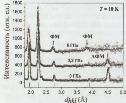
Рис. 8. Участки нейтронных дифракционных спектров \text{La}_{0,5}\text{Ba}_{0,5}\text{CoO}_{2,8} полученные при давлениях 0, 2,2 и 6,0 ГПа и температуре T = 10 К, обработанные по методу Ритвельда. Характерные магнитные пики указаны как АФМ и ФМ. Вертикальными штрихами обозначены рассчитанные положения структурных пиков кубической фазы при нормальном давлении.
