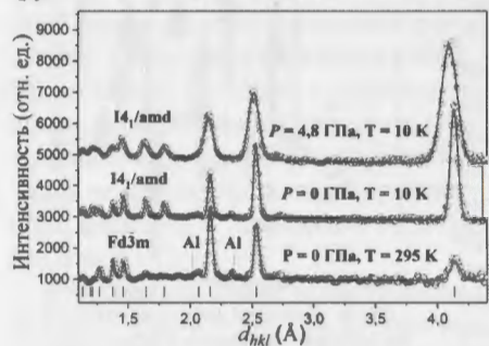
Рис. 14. Участки нейтронных дифракционных спектров \text{HoCo}_2 , полученные при давлениях 0 и 4,8 ГПа, при комнатной и низкой ( T = 10 К) температурах, обработанные по методу Ритвельда. ФМ фаза имеет вклад во все структурные пики спектров при T = 10 К. Вертикальными штрихами внизу обозначены рассчитанные положения структурных пиков при P = 0 ГПа и T = 295 К.
