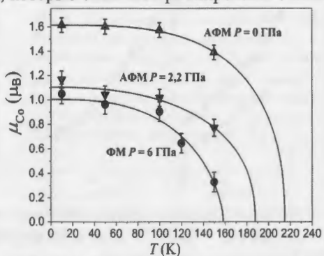
Рис. 10. Температурная зависимость упорядоченных магнитных моментов \text{Co} в \text{La}_{0,5}\text{Ba}_{0,5}\text{CoO}_{2,8} для АФМ и ФМ фаз при различных давлениях. Сплошные линии – интерполяция экспериментальных данных функцией (1).
