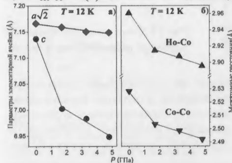
Рис. 15. Барические зависимости параметров элементарной ячейки \text{HoCo}_2 (а) и межатомных расстояний: Ho-Co и Co-Co (б) при T = 12 К. Ошибки не превышают размеров символов. Сплошные линии – линейная интерполяция экспериментальных данных.
