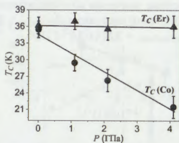
Рис. 23. Зависимости T_C кобальтовой и эрбиевой подрешёток. Сплошные линии – линейная интерполяция экспериментальных данных.
