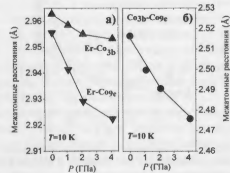
Рис. 20. Барические зависимости межатомных связей \text{Co}_{3b}\text{-Er} , \text{Co}_{9e}\text{-Er} и \text{Co}_{9e}\text{-Co}_{3b} в \text{ErCo}_2 при T = 10 К. Ошибки не превышают размеров символов. Сплошные линии – линейная интерполяция экспериментальных данных.
