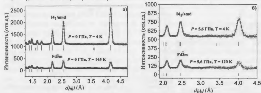
Рис. 11. Участки нейтронных дифракционных спектров \text{DyCo}_2 , полученные при давлениях 0 ГПа и 5,6 ГПа, обработанные по методу Ритвельда. ФМ фаза имеет вклад во все структурные пики спектра при T = 4 \text{ К} . Вертикальными штрихами внизу обозначены рассчитанные положения структурных пиков при T = 290 \text{ К} .
