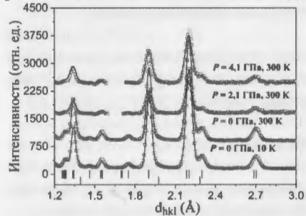
Рис. 1. Участки нейтронных дифракционных спектров \text{La}_{0,8}\text{Ba}_{0,2}\text{CoO}_3 , полученные при давлениях 0, 2,1 и 4,1 ГПа, при комнатной и низкой (для P = 0 \text{ ГПа} , T = 10 \text{ К} ) температурах, обработанные по методу Ритвельда. Вырезанные участки на спектрах между 1.6 и 1.7 Å соответствуют сапфировым пикам от камеры высокого давления.
